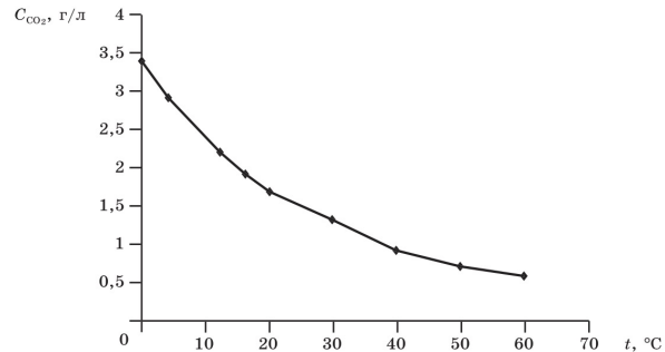
Рис. 2. Зависимость растворимости углекислого газа в воде от температуры при нормальном атмосферном давлении
